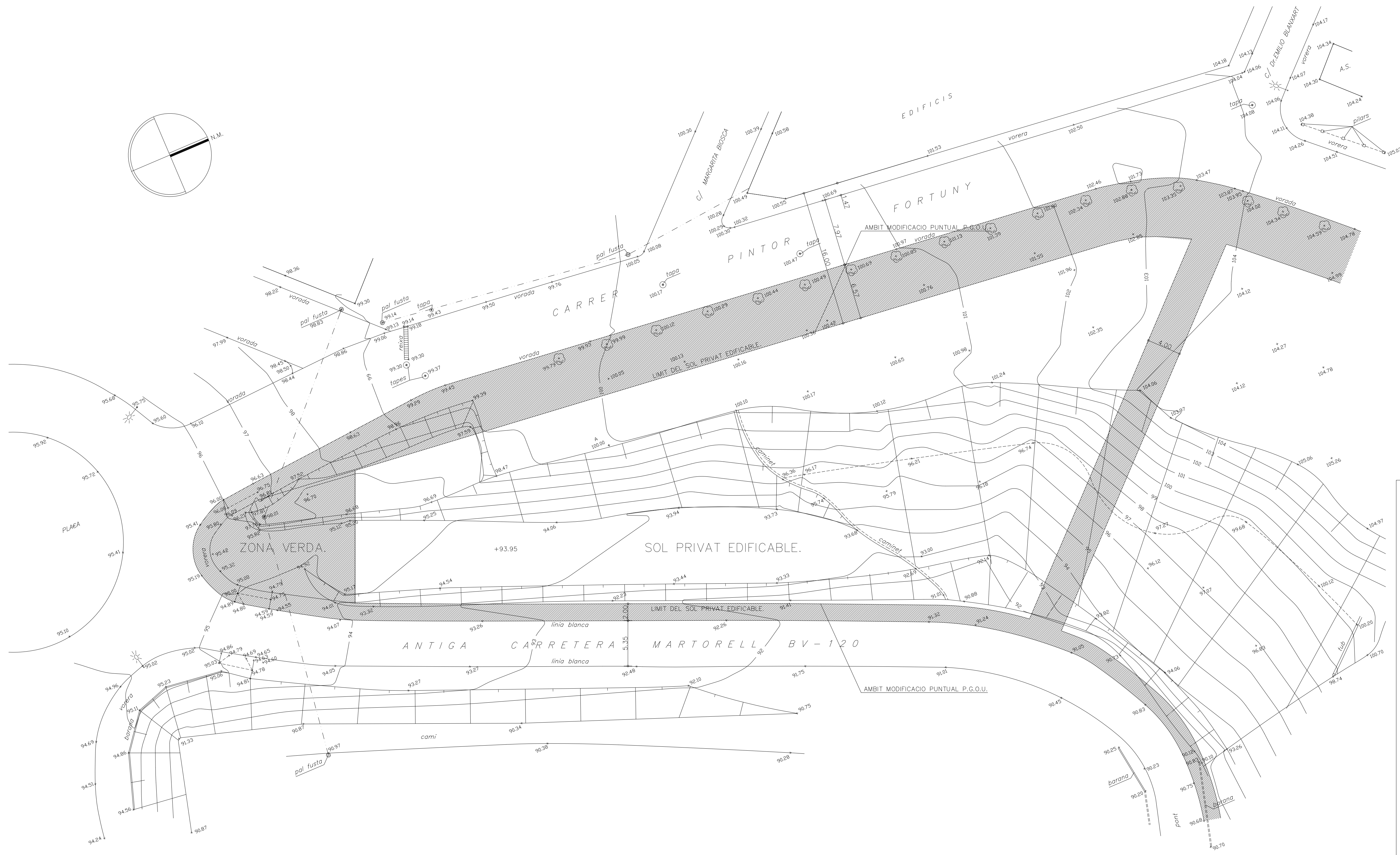
TOPOGRAFIC ESTAT ACTUAL. AMBIT MODIFICACIO. ESCALA 1:200 SUPERFICIE SOL PRIVAT EDIFICABLE = 2619.40 m2
