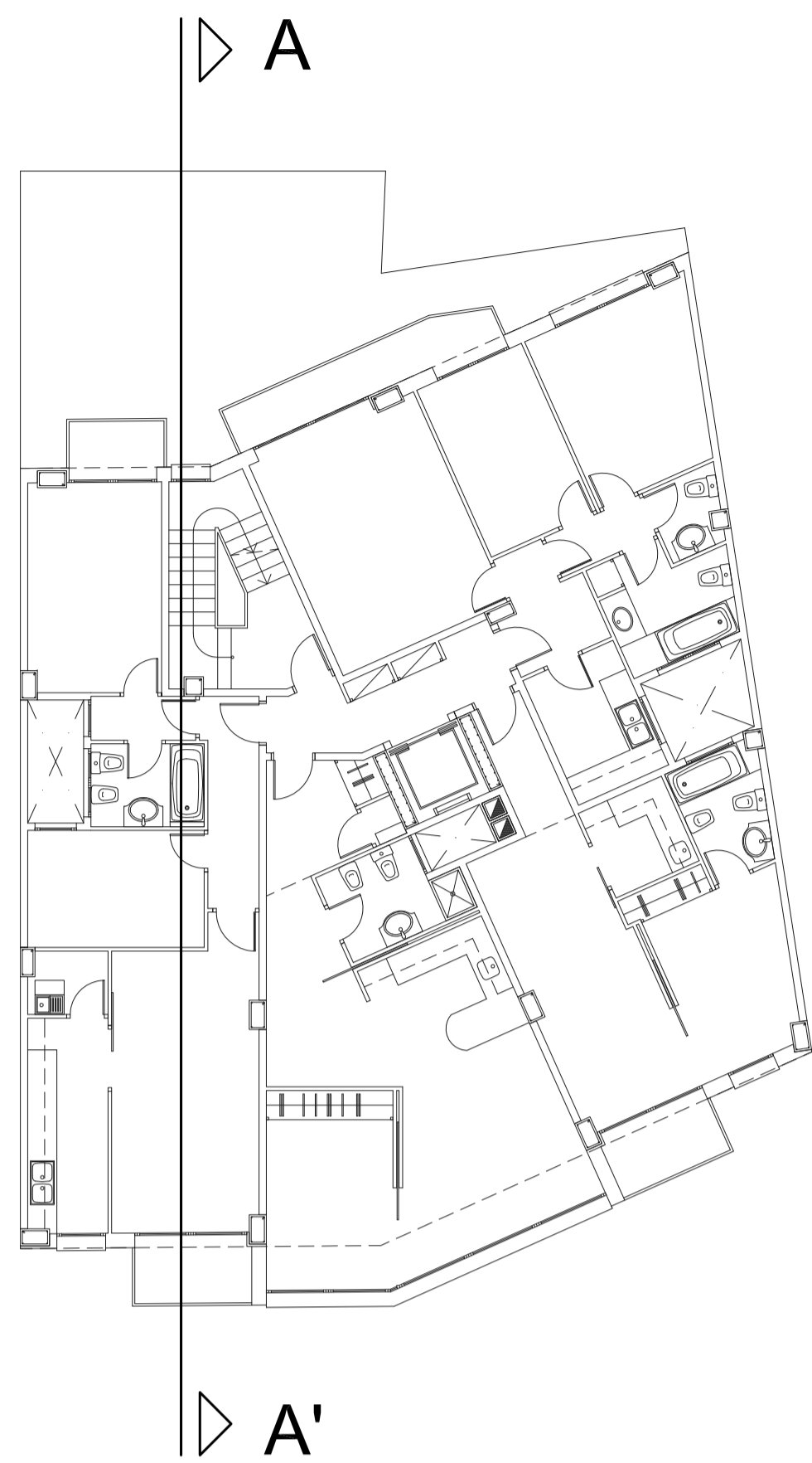
PLANTA ESQUEMA.
