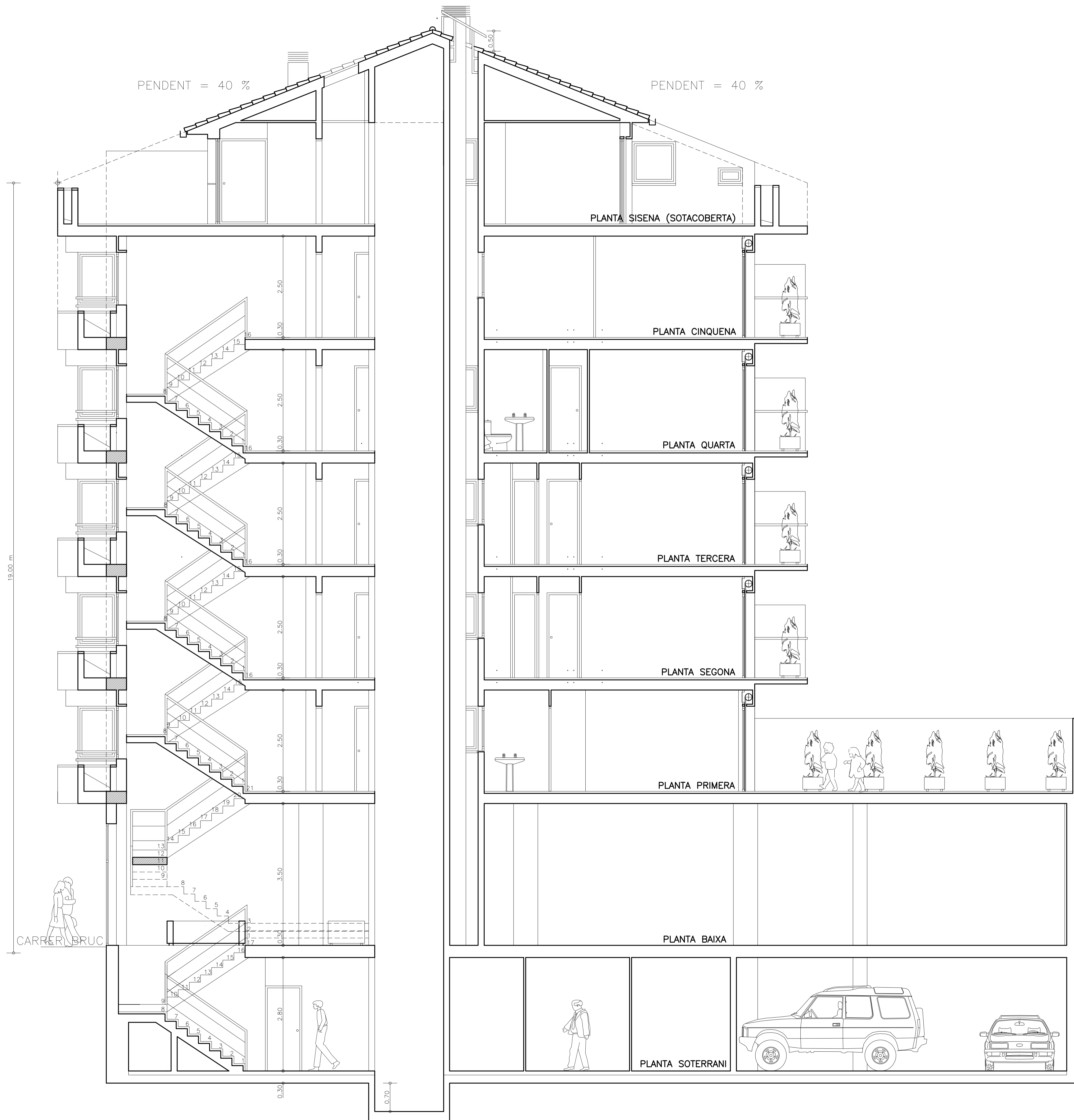
SECCIO TRANSVERSAL AA'
