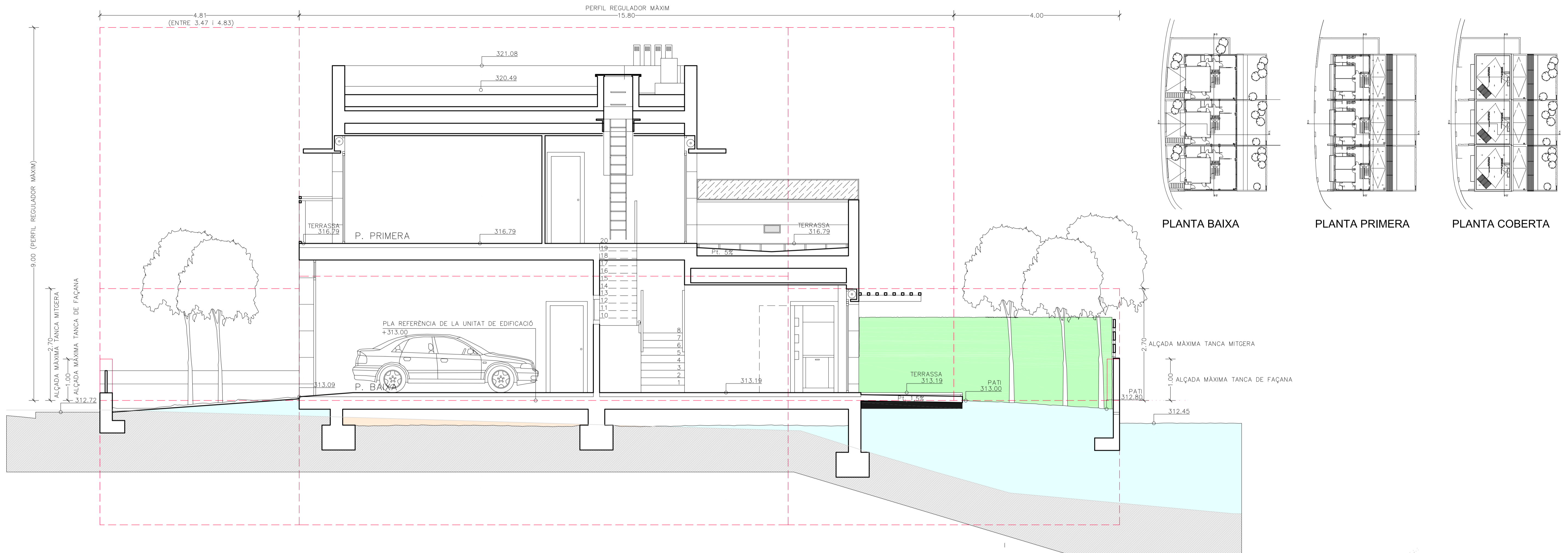
SECCIÓ A-A' ESCALA 1:50
