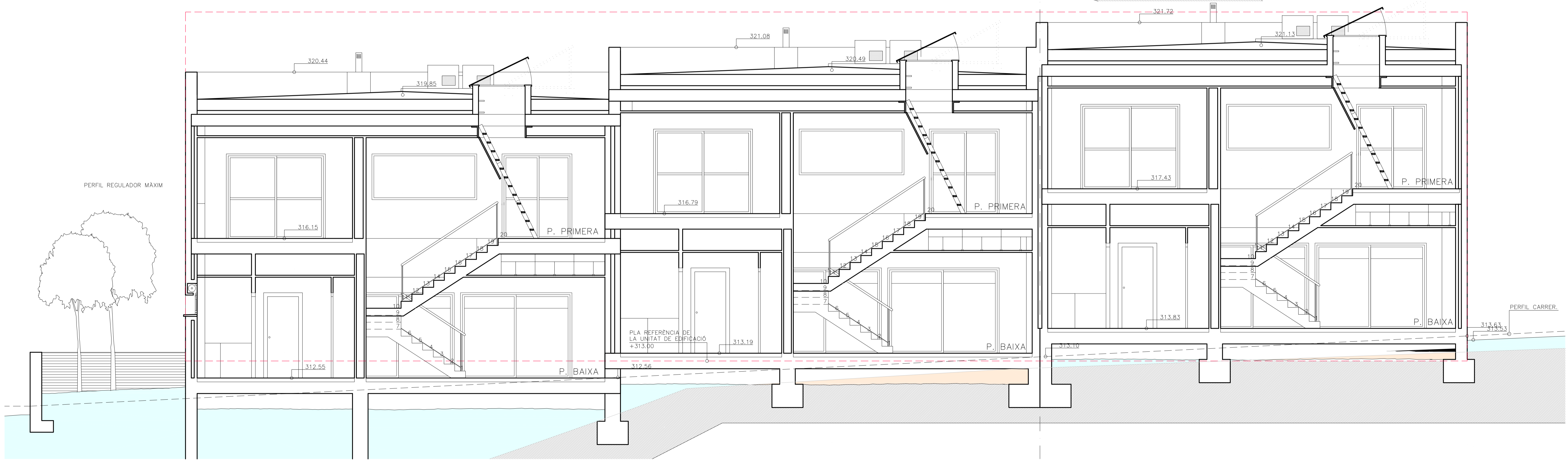
SECCIÓ A-A' ESCALA 1:50
