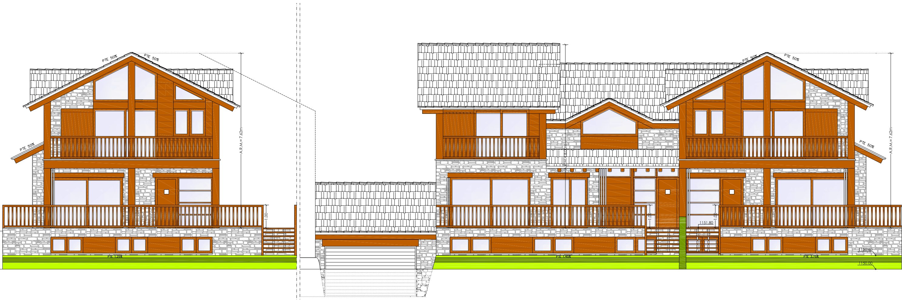
FAÇANA PRINCIPAL CONJUNT PARCEL.LA 8
