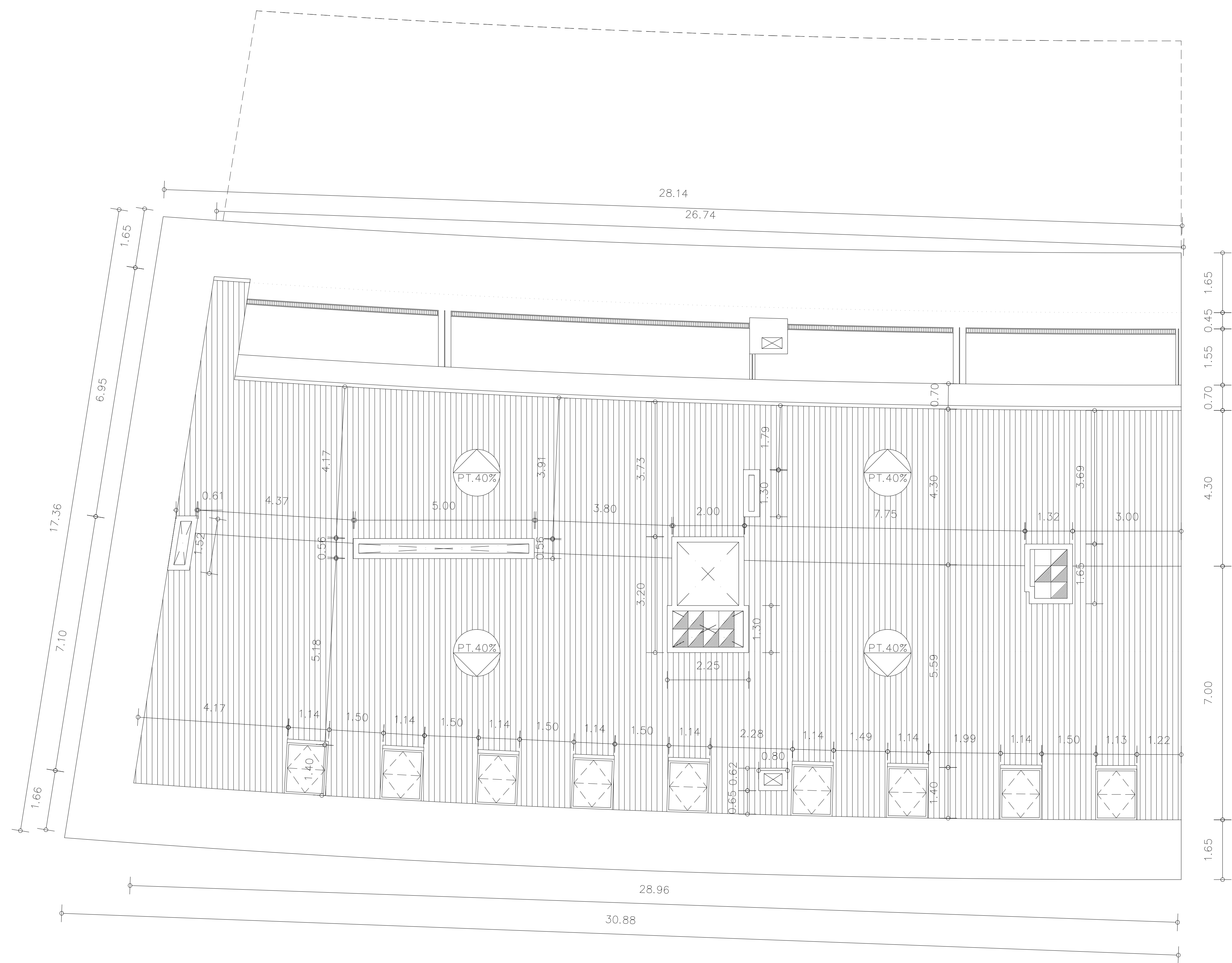
PLANTA COBERTA.
